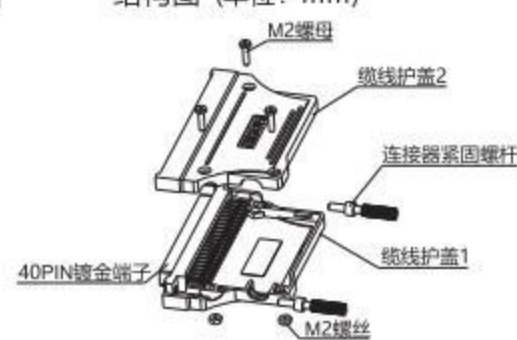
结构图 (单位: mm)
