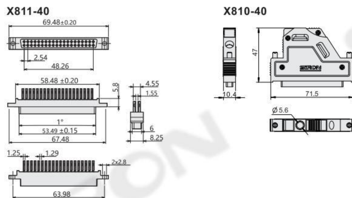
结构图 (单位: mm)
